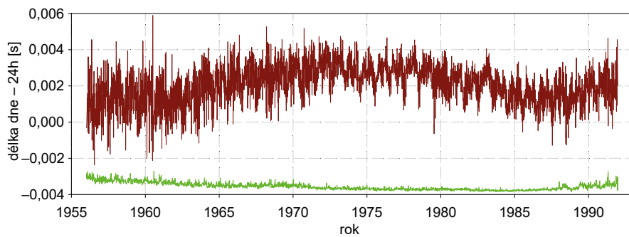
Obr. 16 Odchylyky délky dne od 24 hodin (v časových sekundách), odvozené z pozorování optickou astrometrií v letech 1956–1992. J. Vondrák, C. Ron, V. Štefka: Acta Geodyn. Geomat. 7 , 245–251 (2010).
